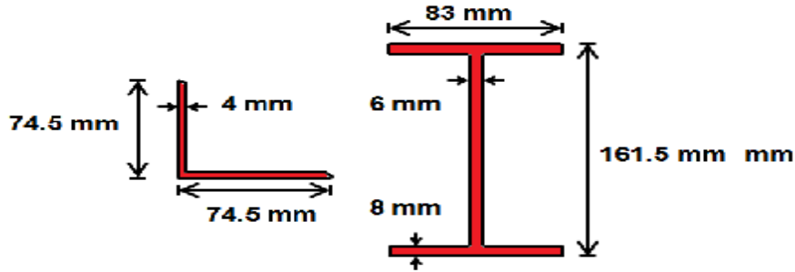
شكل رقم (4) مقاطع الحديد
