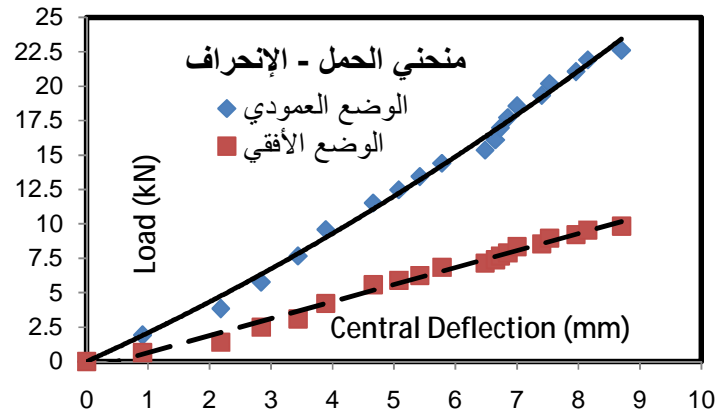
شكل رقم (13) منحني الحمل – الإنحراف
