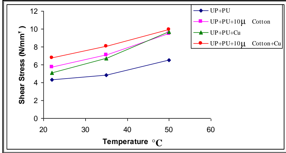
الشكل (9) يوضح التغير في إجهاد قص ( \tau_{max} ) للانحناء ودرجات حرارية مختلفة لعينات المترابكات البوليمرية.
