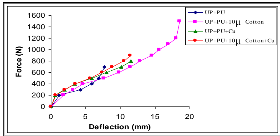
الشكل (6) يوضح العلاقة بين الحمل المسلط مع مقدار الانحراف الحاصل في إختبار متانة الانحناء للعينات المترابطة عند درجة حرارة (50±4 °C).
