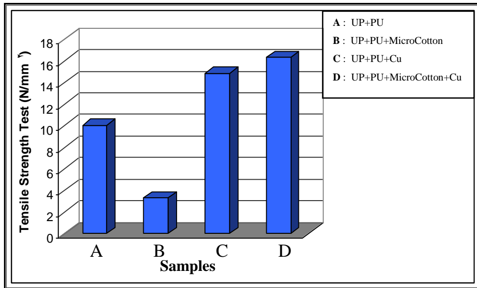
الشكل (10) يوضح تغير قيم متانة الشد لجميع نماذج الخلطات البوليمرية المترابكة في البحث.
